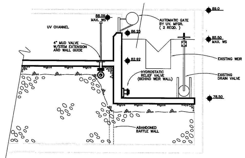
5 UV BASIN SECTION SCALE: 1" = 1' - 0"
