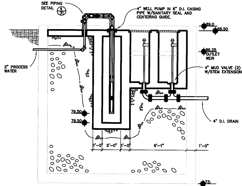
2 UV BASIN SECTION SCALE: 1" = 1' - 0"
