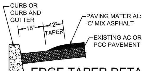
EDGE TAPER DETAIL
