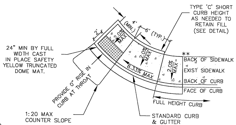
6 ADA RAMP OPTIONS N.T.S.
