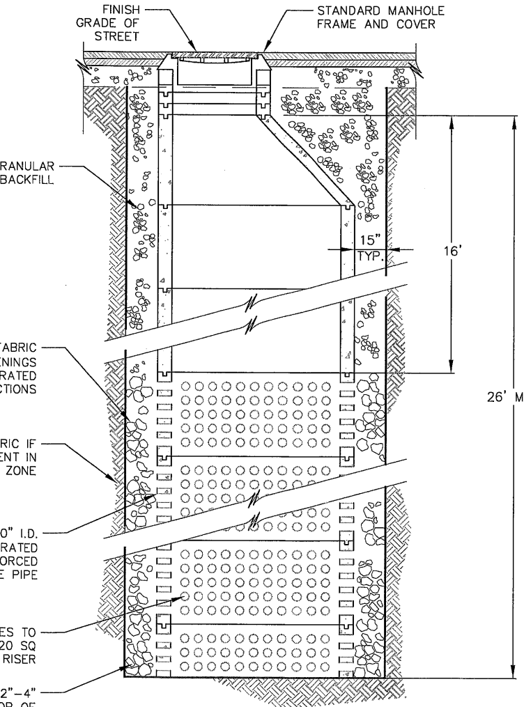
7 STANDARD DRYWELL N.T.S.
