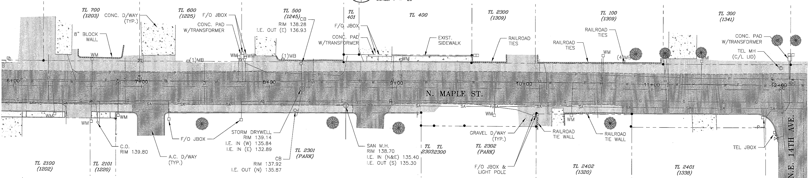
STA 6+00 - STA 12+00 N. MAPLE STREET - PLAN SCALE: 1" = 20'
